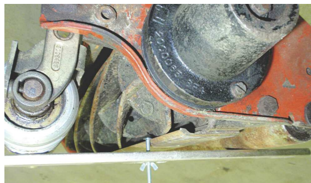
Ukázka měření a nastavení výšky sečení u vřetenové sekačky pomocí měřky se šroubem. Výška sečení je pak měřena posuvným měřítkem mezi měrkou a hlavičkou šroubu.
